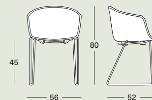
P 7050, U 7051 Slitta / Sled base
