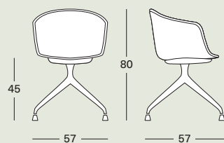
P 7630, U 7631 Trespolo con piedini, girevole / Trestle base, swivel
